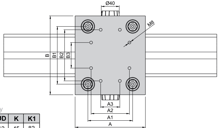
Blok Yatak Gövde / Roller Black Guide Body
