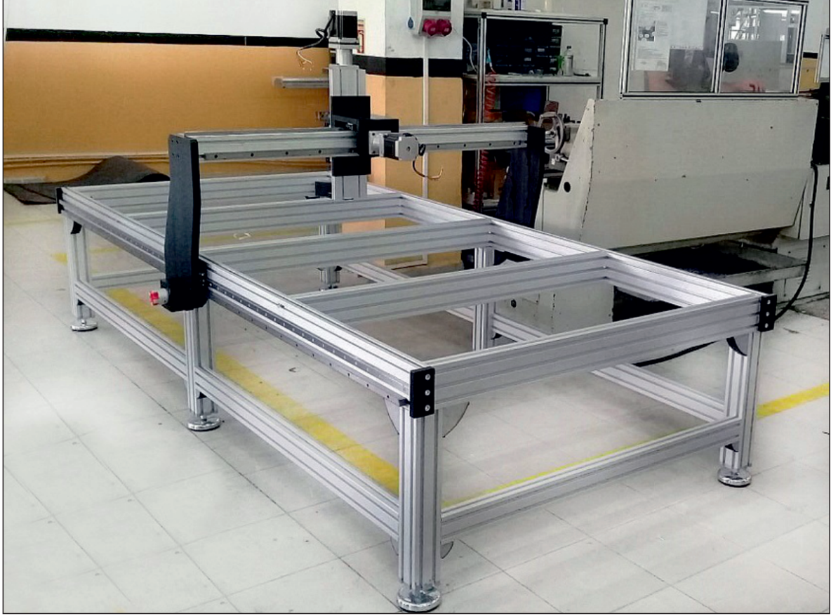
Barkodlama Otomasyonu / Barcode Otomation
