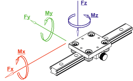
Yükleme Değerleri / Upload Values
