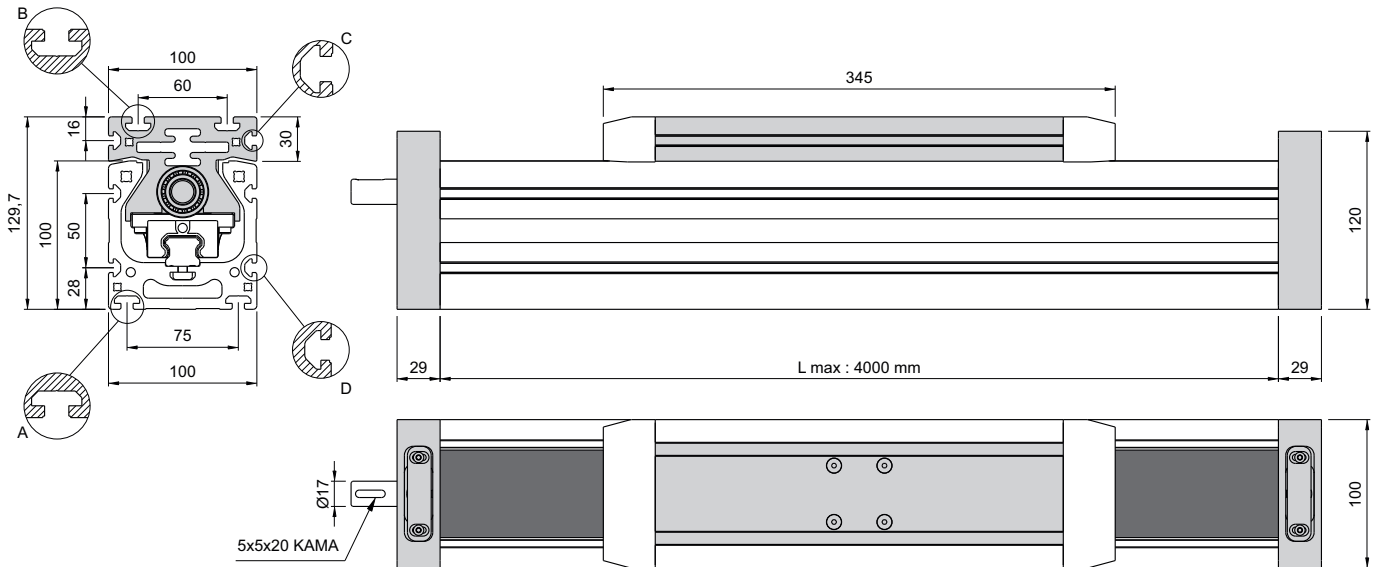
A (M8 KANAL DETAY) B (M8 KANAL DETAY) C (M6 KANAL DETAY) D (M6 KANAL DETAY)
