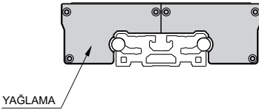
Blok Yatak Gövde / Roller Block Guide Body
