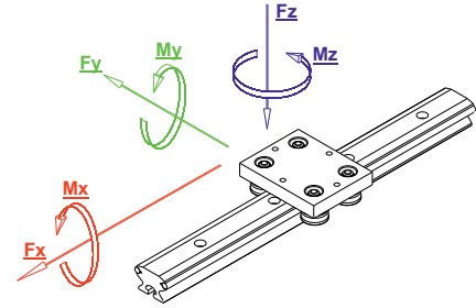
Yüklemeye Değerleri / Upload Values
