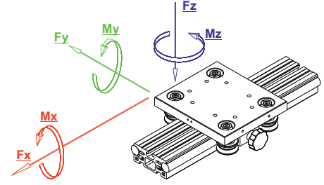
Yüklemeye Değerleri / Upload Values
