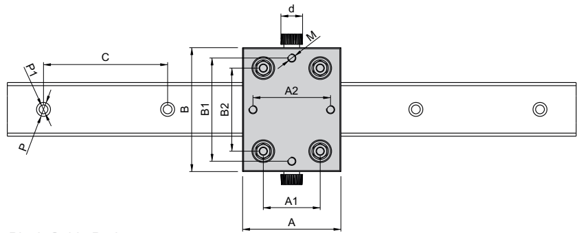
Blok Yatak Gövde / Roller Block Guide Body
