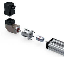
Akuplasyon Çeşitleri / Types of Acupulation
