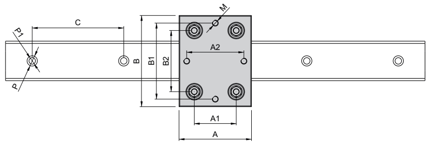
Blok Yatak Gövde / Roller Block Guide Body
